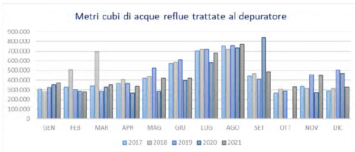
Figura 25. Andamento mensile dei liquami trattati dal Depuratore di Cervia (Servizio Qualità HERA)
