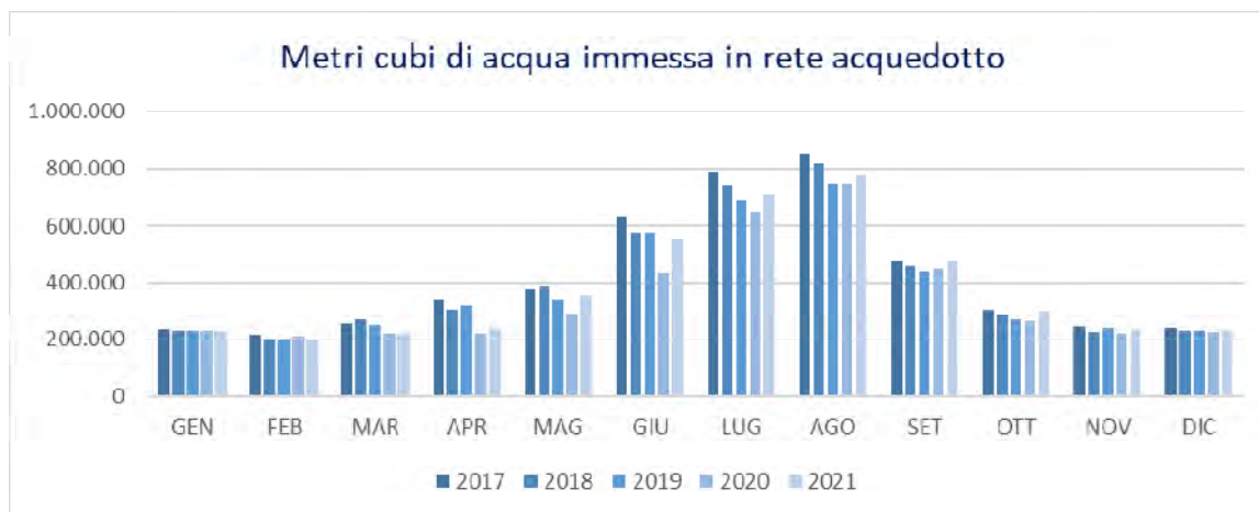
Figura 23. Andamento mensile della distribuzione di acqua potabile a Cervia (dati HERA)
